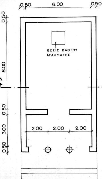
ΚΑΤΟΨΙΣ ΚΛ. 1:100
