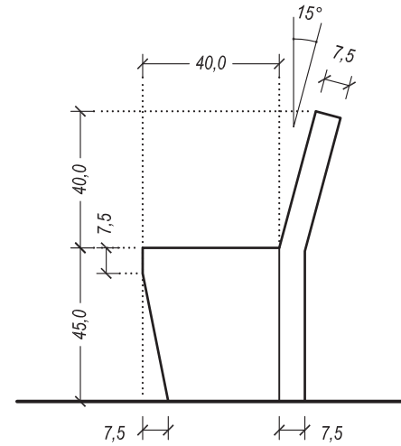
ΠΛΑΓΙΑ ΟΨΗ
