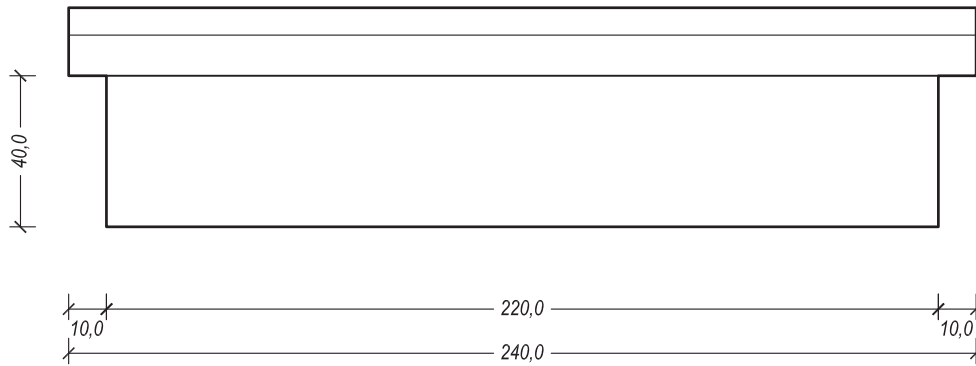
ΚΑΤΟΨΗ
