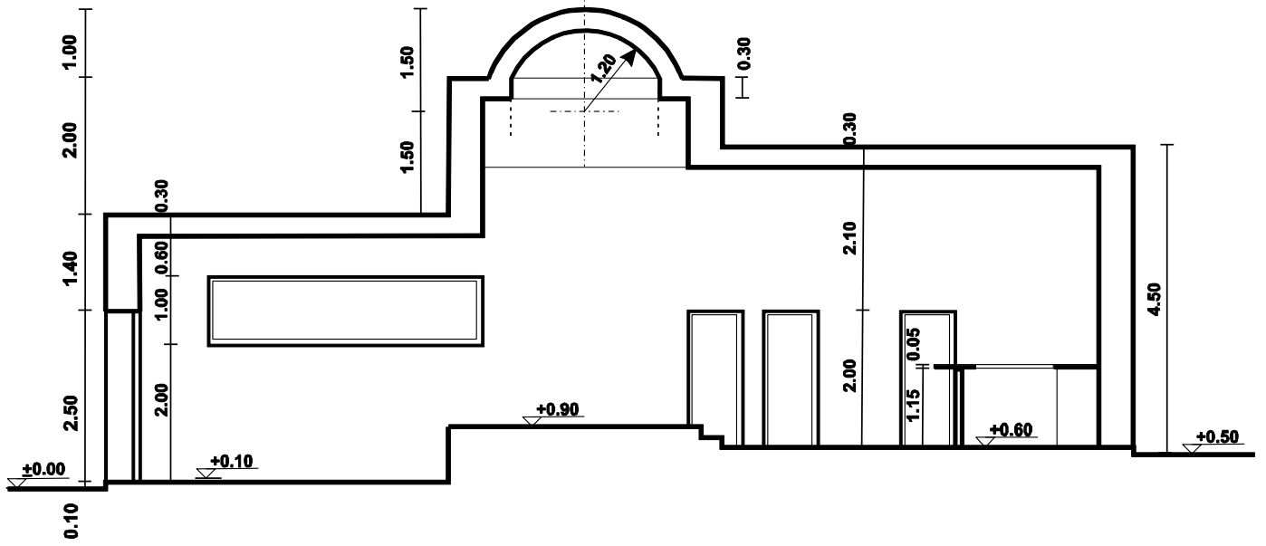
ΤΟΜΗ Α-Α
